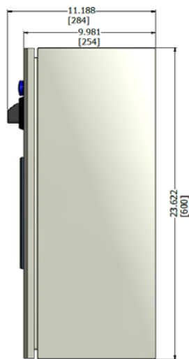
Side (NEMA 1/NEMA 4X)
